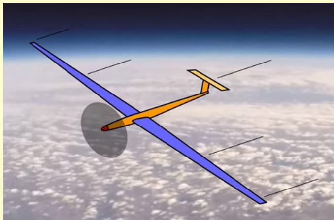
Fig. 2 - Drone électro solaire stratosphérique CMI ATE.
